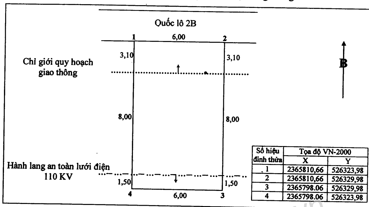
Hình 1 – Sơ đồ thửa đất có đầy đủ các nội dung thông tin
