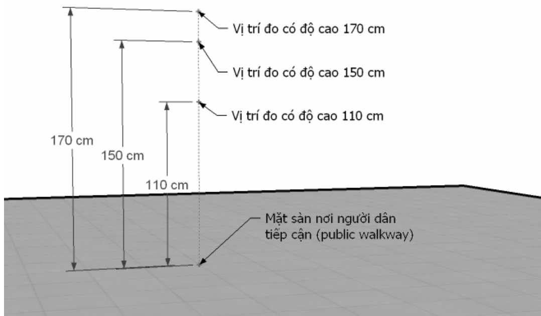
Hình 2. Vị trí đo tại từng điểm đo
