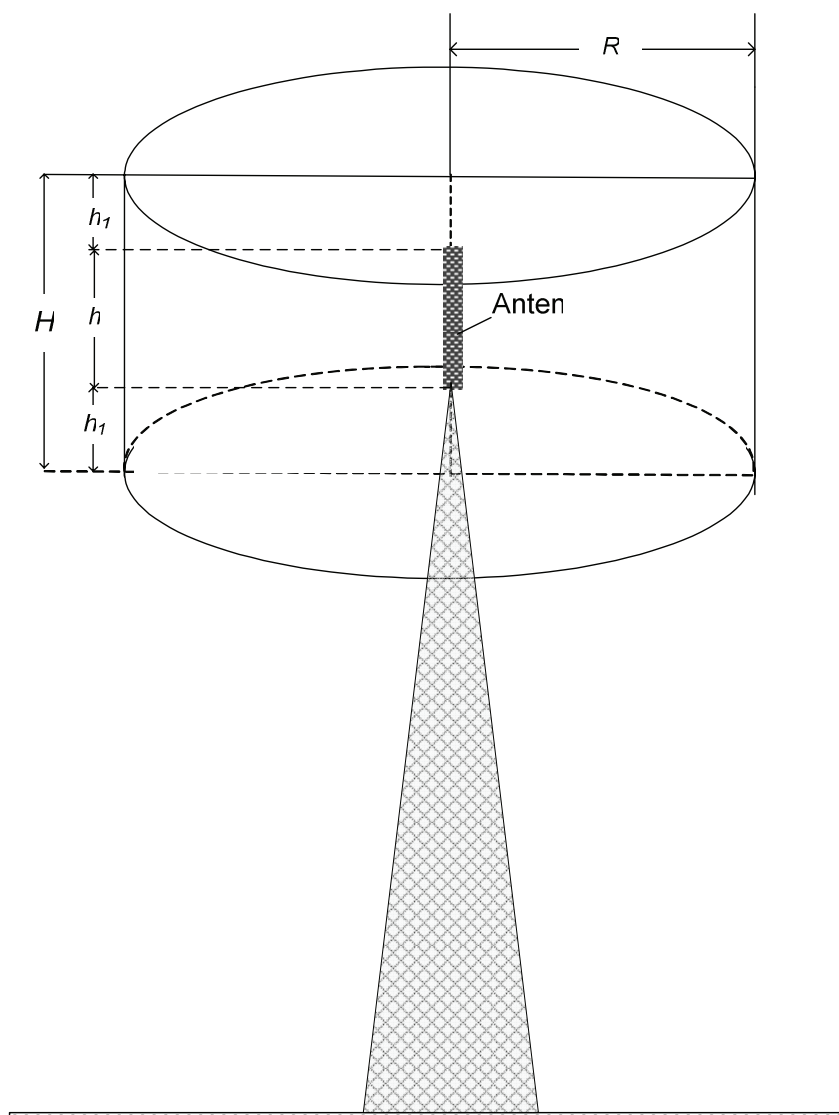
Hình A.3. Minh họa vùng tuân thủ của đài phát thanh, truyền hình sử dụng anten đẳng hướng
