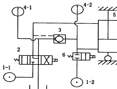
Hình 33: Sơ đồ nguyên lý thử nghiệm van một chiều điều khiển thủy lực
