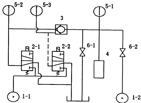
Hình 32: Sơ đồ nguyên lý thử nghiệm van một chiều điều khiển thủy lực
