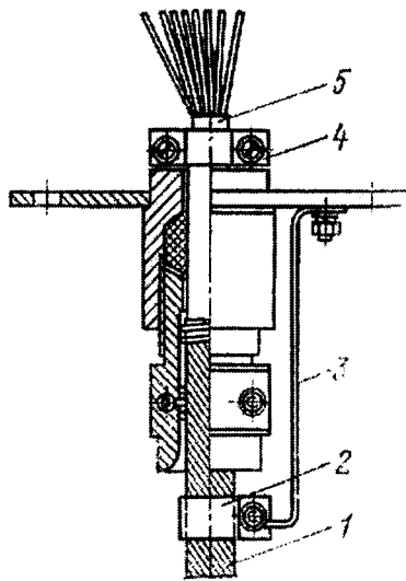
Hình 21 Phụ lục IV - Sơ đồ đấu tiếp đất cho cáp kiểm tra vỏ bọc chì
