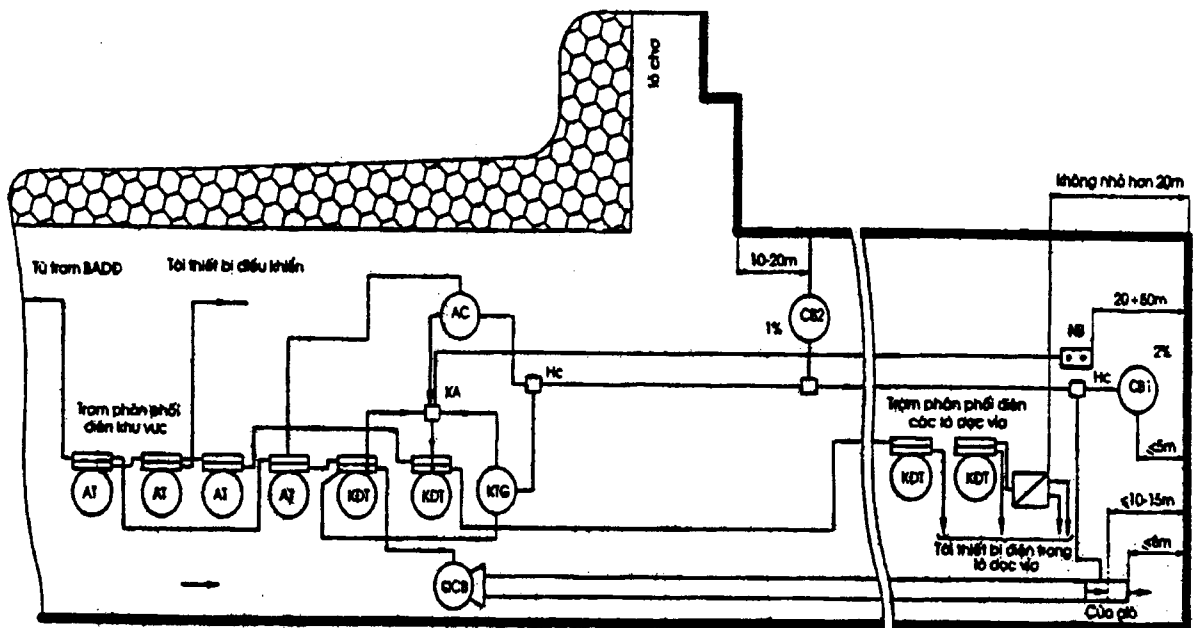
Hình 1 Phụ lục IV - Sơ đồ cung cấp điện và bố trí thiết bị khi đào thương
