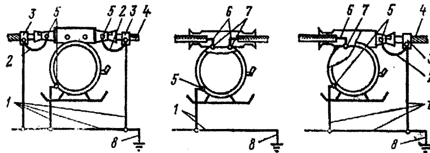
Hình 15 Phụ lục IV - Sơ đồ tiếp đất cho một số thiết bị điện
