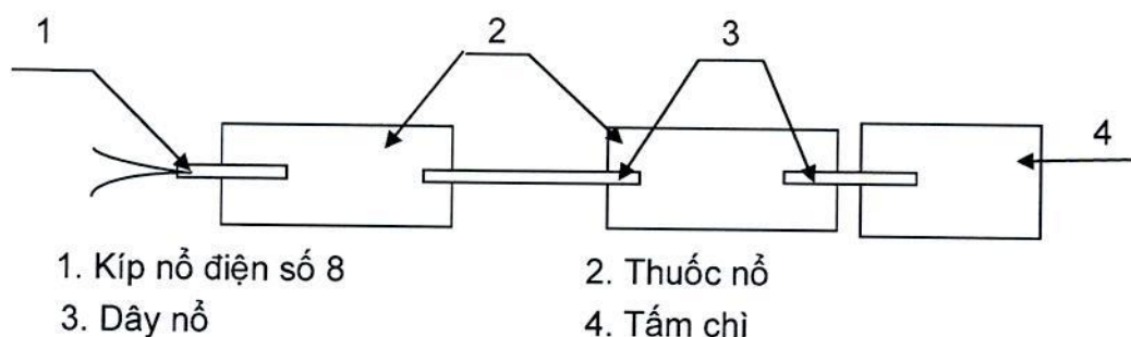
Hình 2 - Sơ đồ xác định khả năng chịu nước
