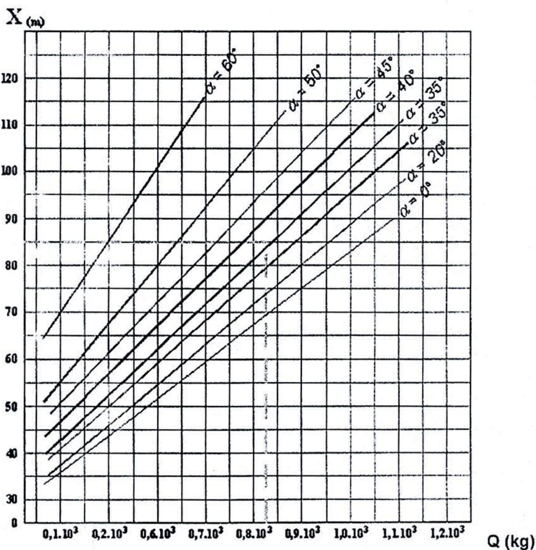
Biểu đồ xác định chiều dài dây cáp X1 khi không có con lăn đỡ
