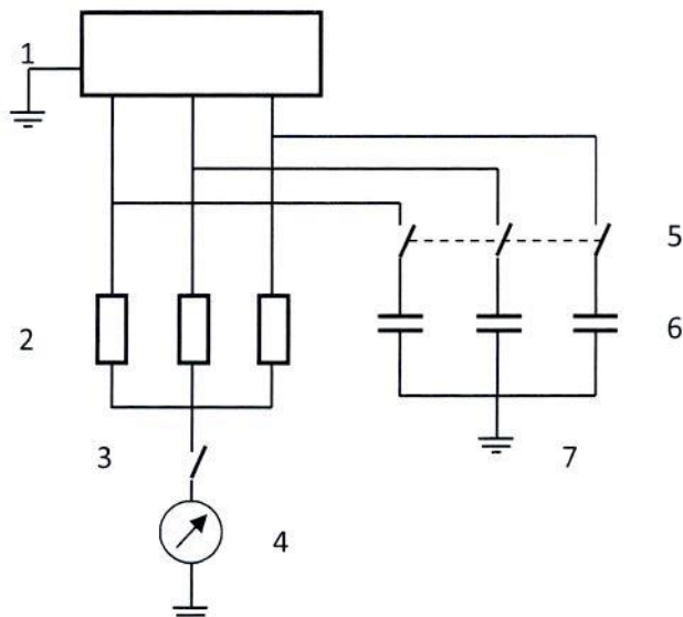
Hình 10. Sơ đồ mô phỏng thử nghiệm rò 3 pha đối xứng
