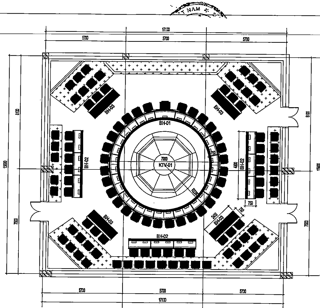
MẶT BẰNG NỘI THẤT PHÒNG HỢP BỘ XÂY DỰNG TỔNG SỐ GHẾ : 115 GHẾ NGỒI
