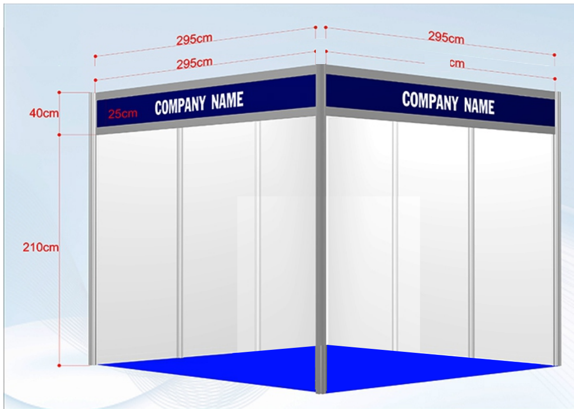
KÍCH THƯỚC GIAN HÀNG TIÊU CHUẨN
