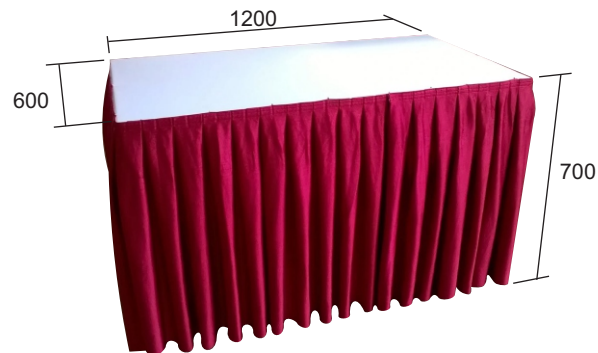
BÀN CÓ KHĂN PHỦ VÀ QUẦY ĐÓ (SỐ LƯỢNG: 1 CHIẾC/1 GIAN)
